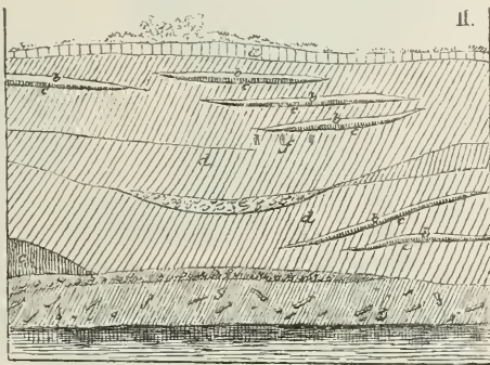
21. sz. A tőszegi terrassara-halom átmetszete, a, c, c a szénrel kevert és agyaggal (A, B, B) váltakozó rétegek. Comptes-Rendus de Budapest II. vol. I-ière partie 22. I. után.
